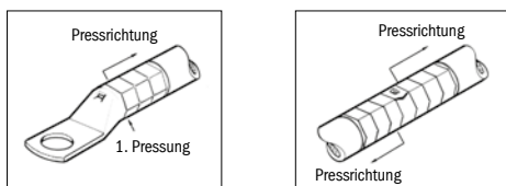
Kerb-/Rohrkabelschuhe
